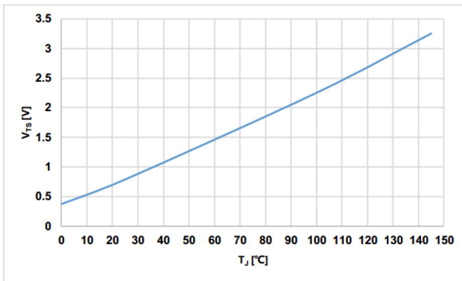
图 5: HVIC 温度检测输出温度—电压曲线
